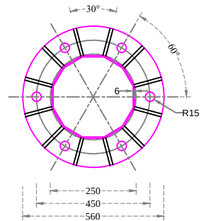
CHI TIẾT BÍCH TRỤ TL 1/20
